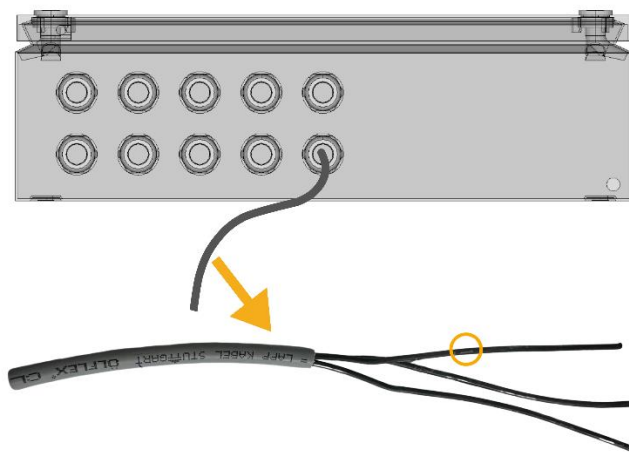
Aanzicht achterzijde regelkast
